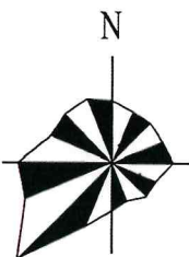
风玫瑰图
